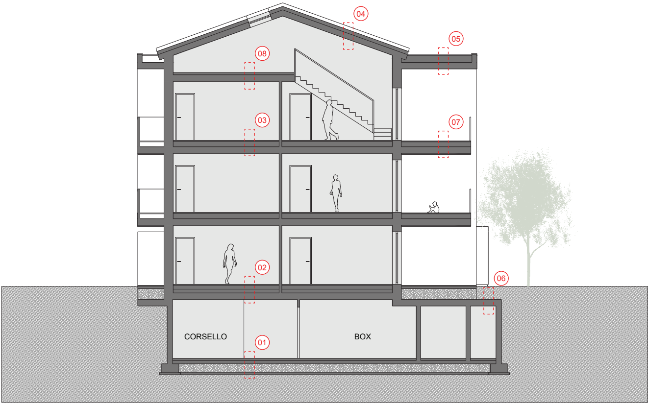
SEZIONE DETTAGLIO SOLAI
